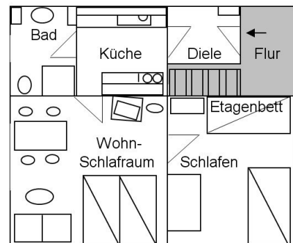
Wohnung 6 Obergeschoss
